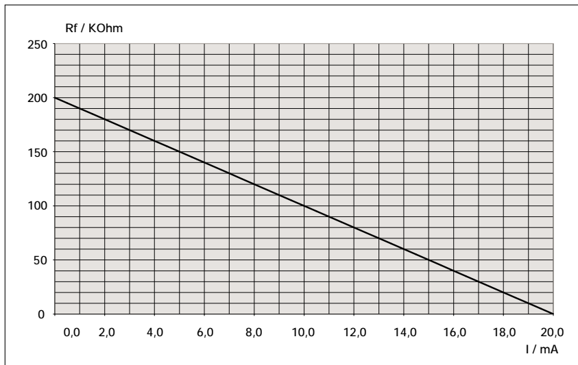
Diagramm: Stromausgang 0 ... 20 mA
